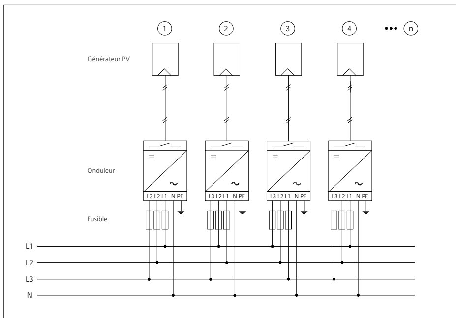
Figure 8.3 : Raccordement côté réseau sur des installations comportant plusieurs onduleurs
