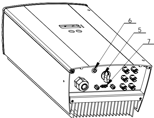
Figure 4.6 : Partie inférieure du Powador
