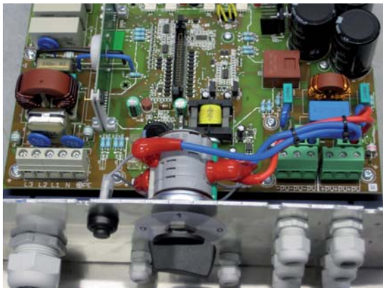
Figure 6.3 : Compartiment de raccordement du Powador
