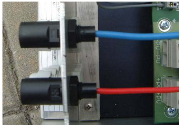
Figure 6.4 : Montage des douilles Tyco
