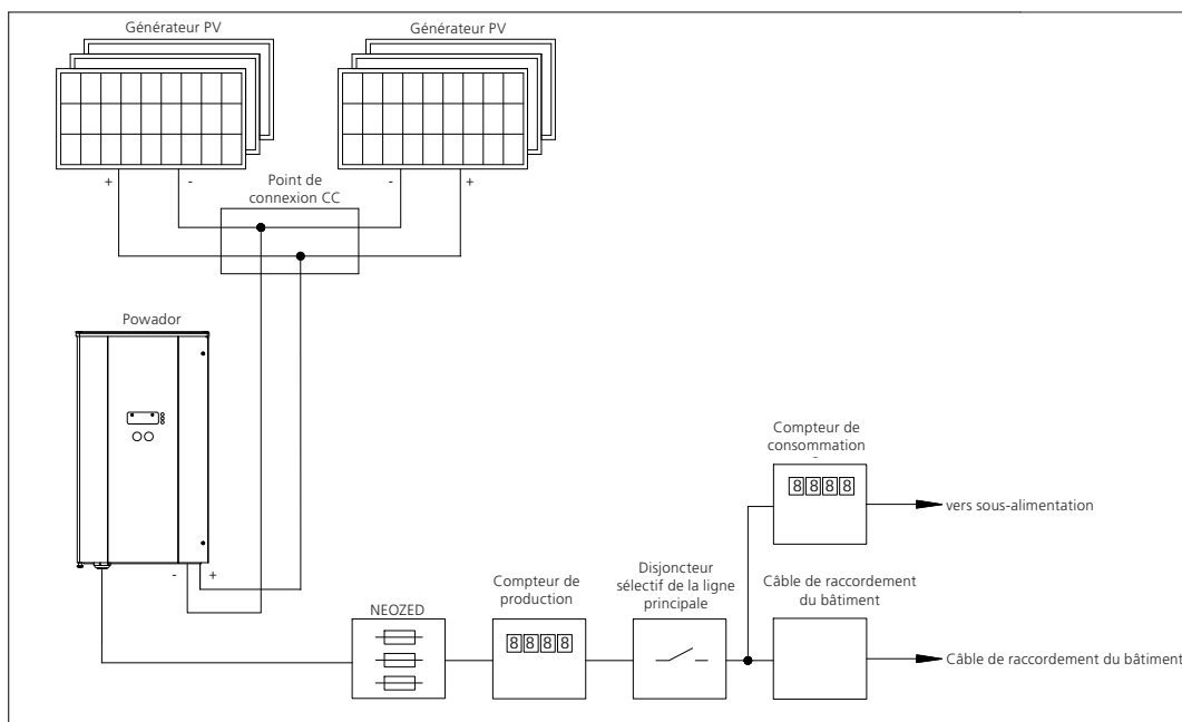
Figure 8.1 Schéma de connexion unipolaire pour une installation équipée d'un onduleur
