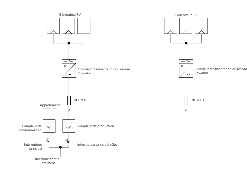
Figure 8.2 Schéma de connexion unipolaire pour une installation équipée de 2 onduleurs
