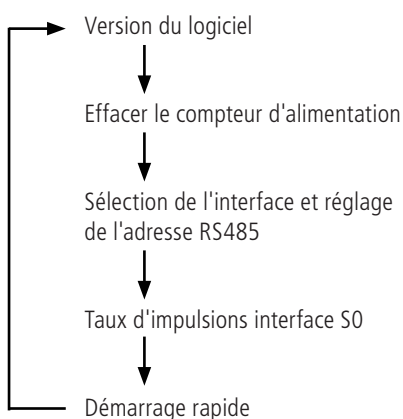
Figure 4.5 : Menu mode de réglage
