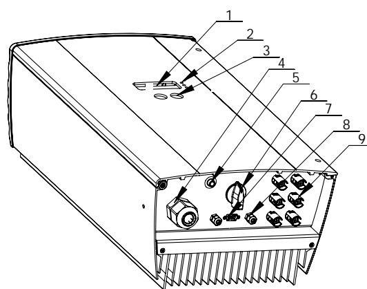
Figure 4.1 : Aperçu du Powador
