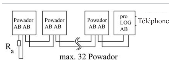
Figure 6.8 : Plan de raccordement de l'interface RS485
